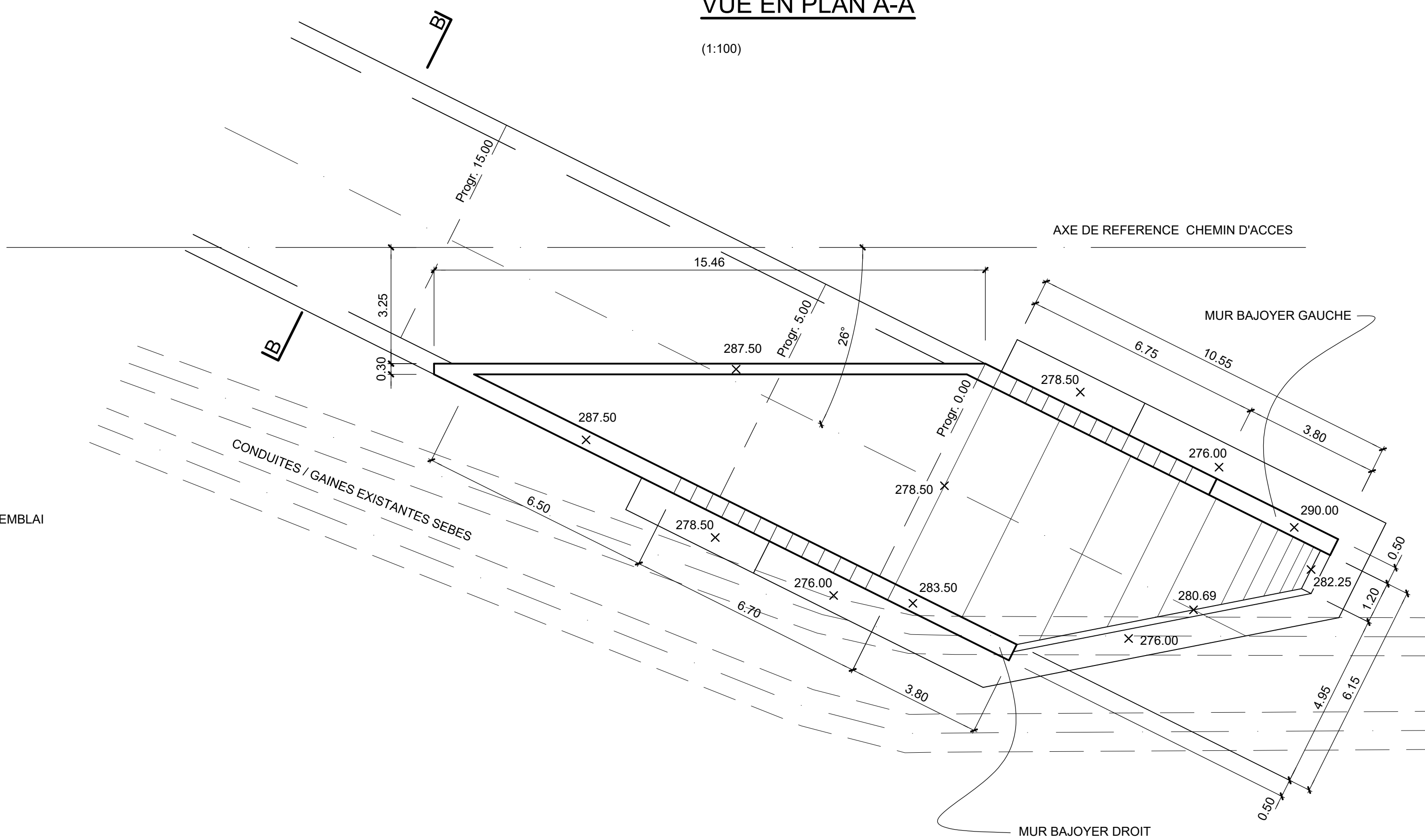
VUE EN PLAN A-A (1:100)
