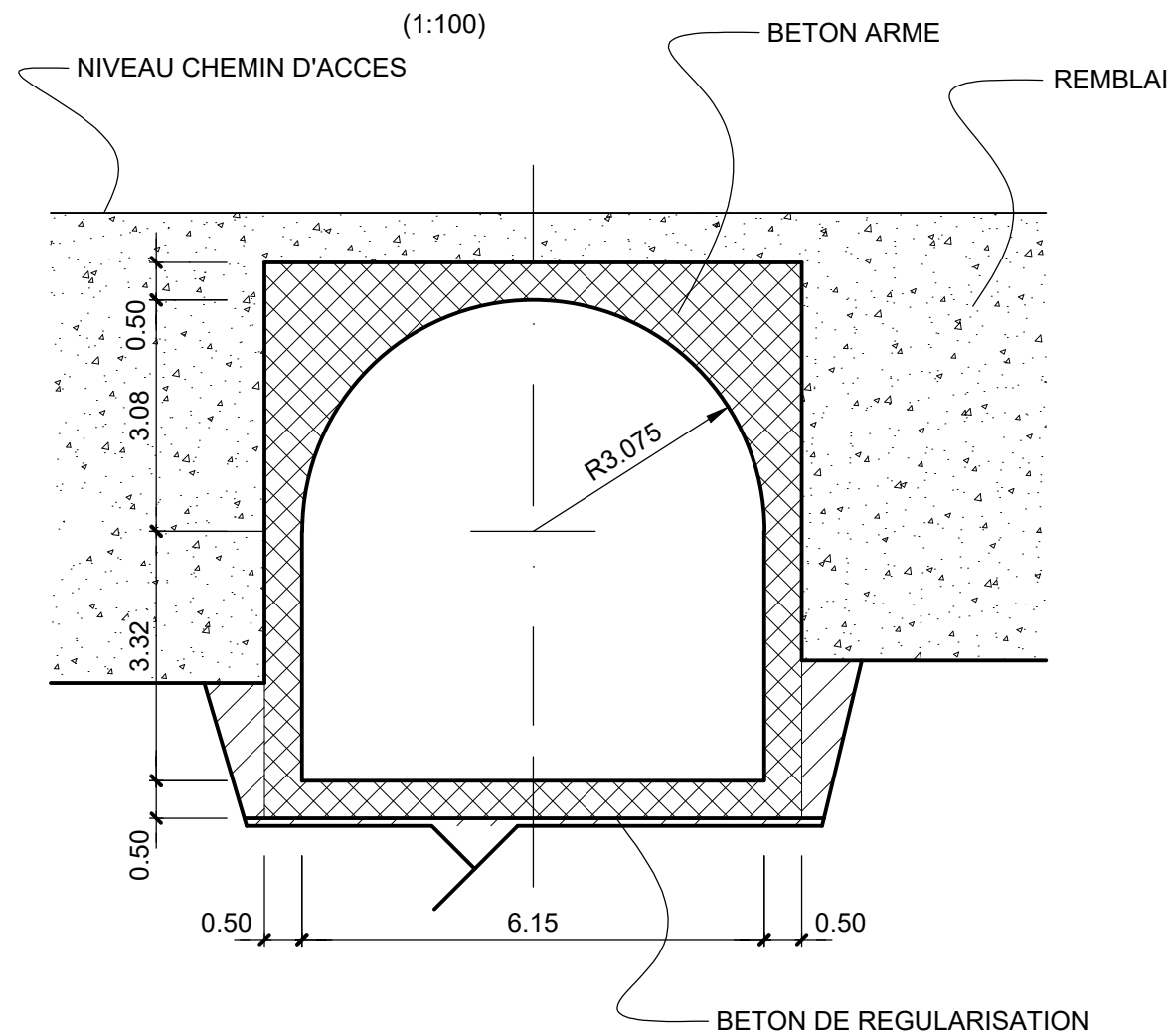
COUPE B-B (1:100)
